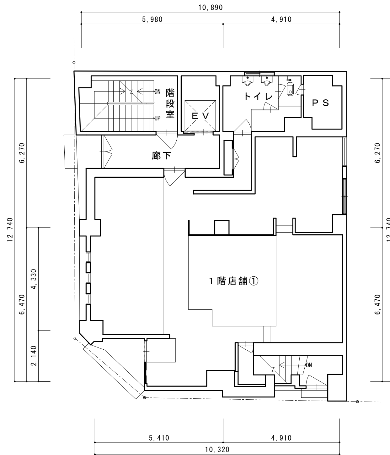
1 F 平面図
