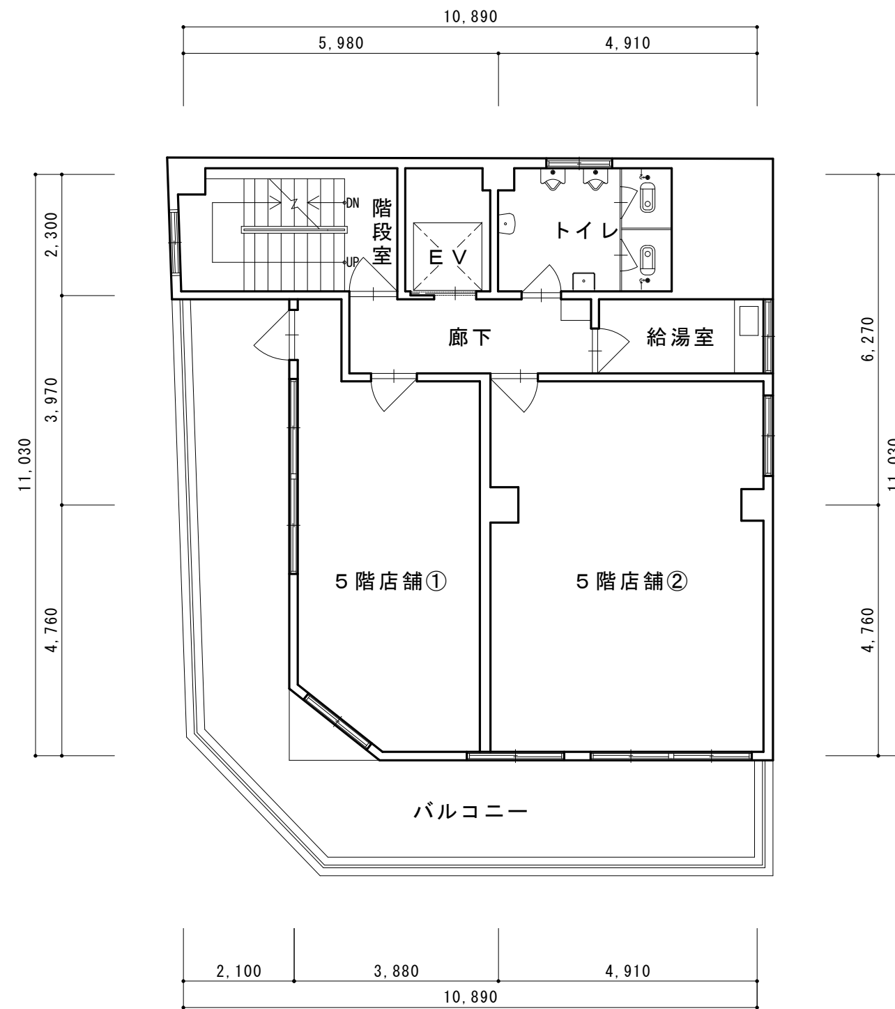
5 F 平面図
