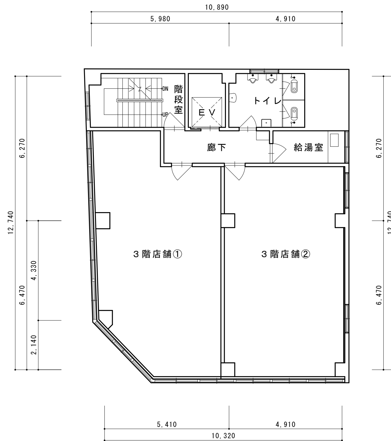
3 F 平面図
