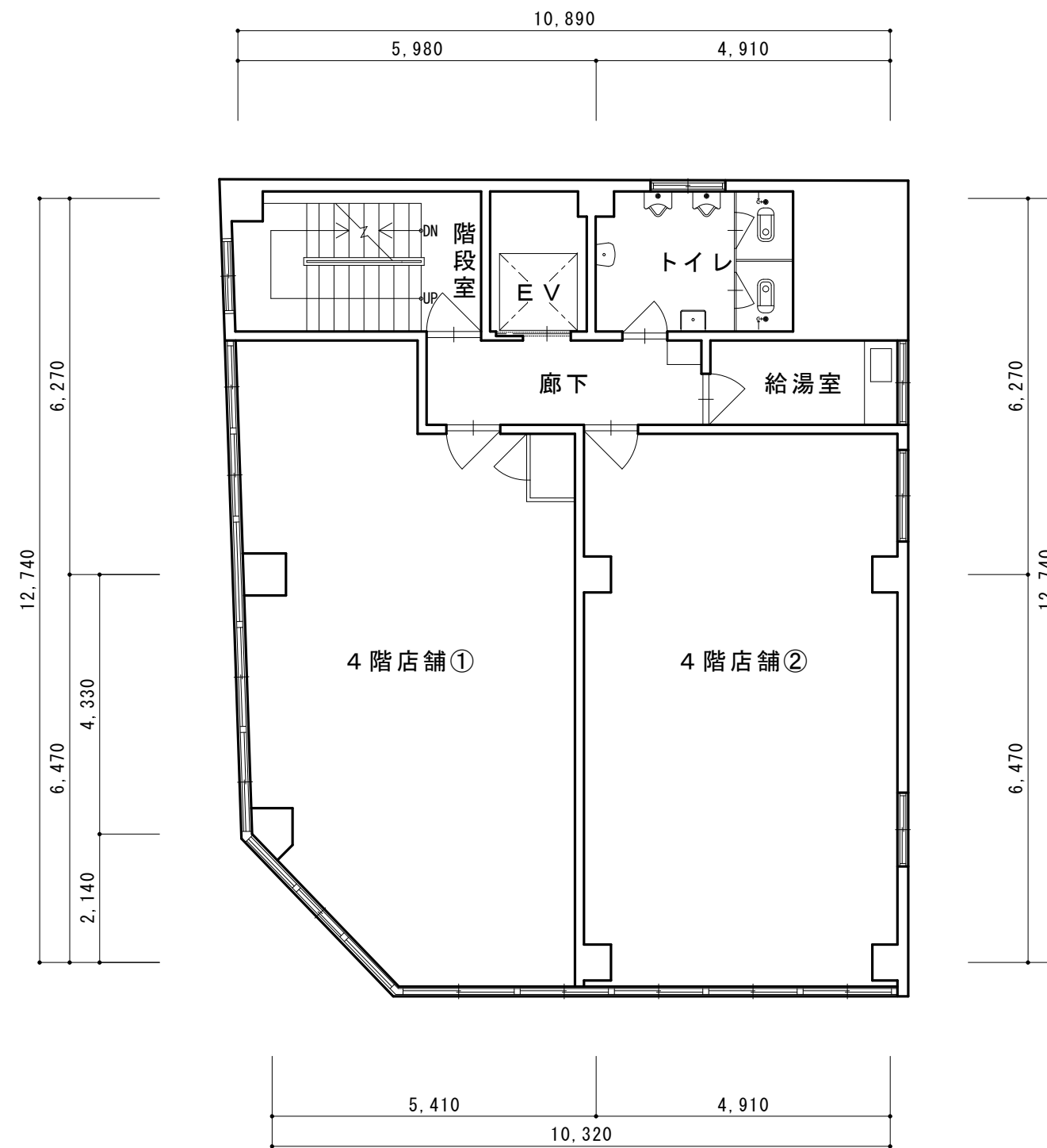
4 F 平面図
