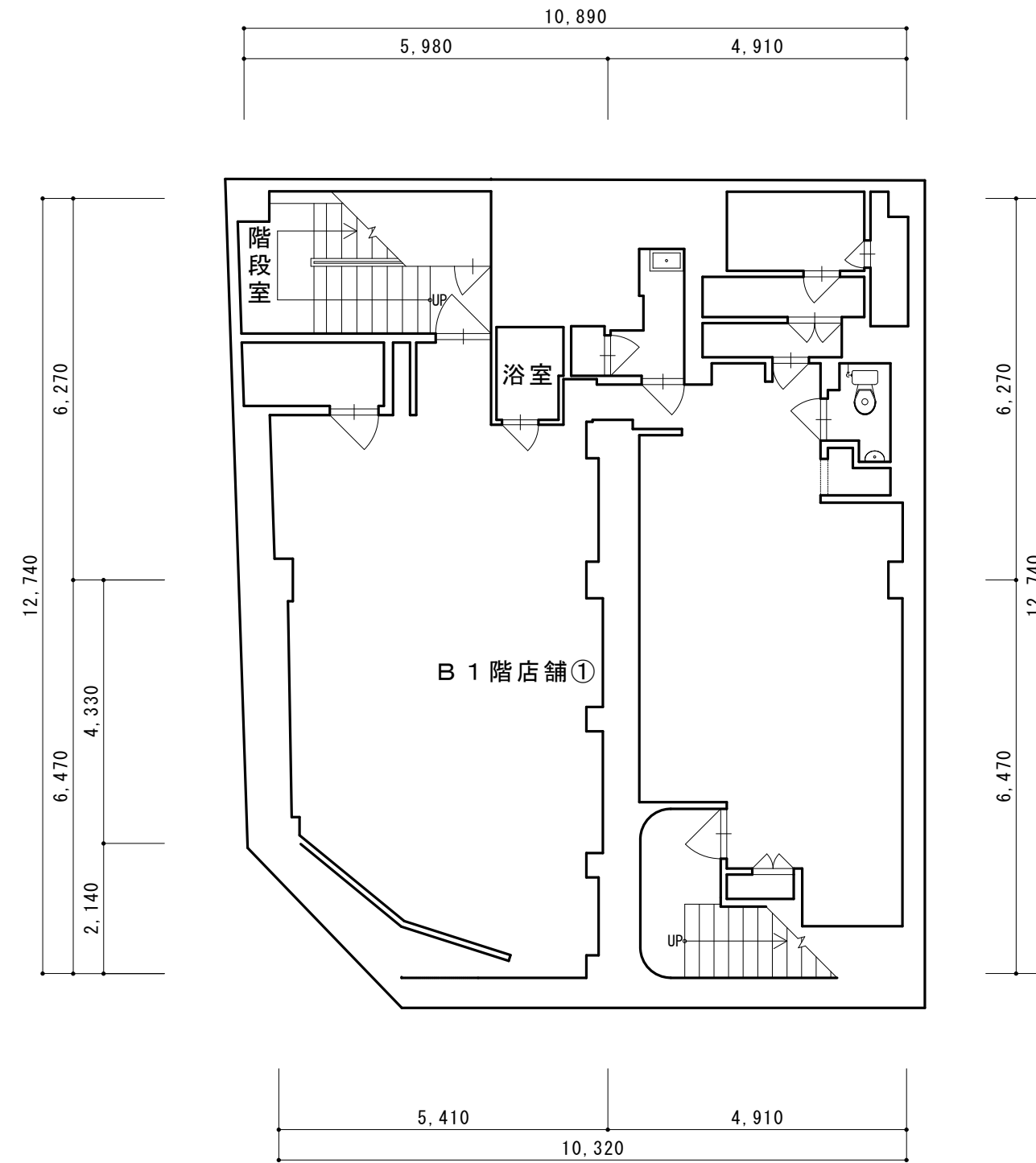
B 1 F 平面図
