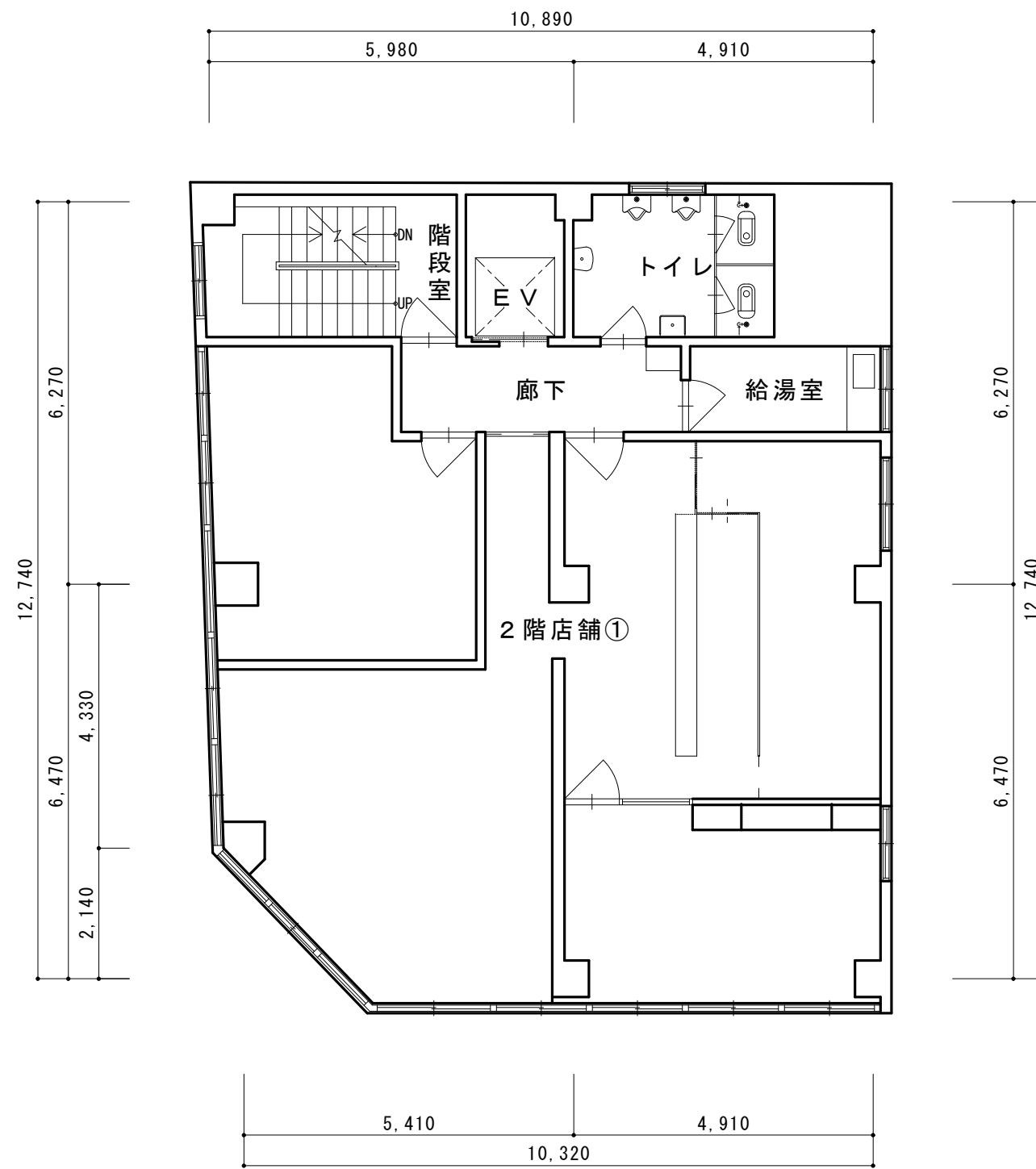
2 F 平面図
