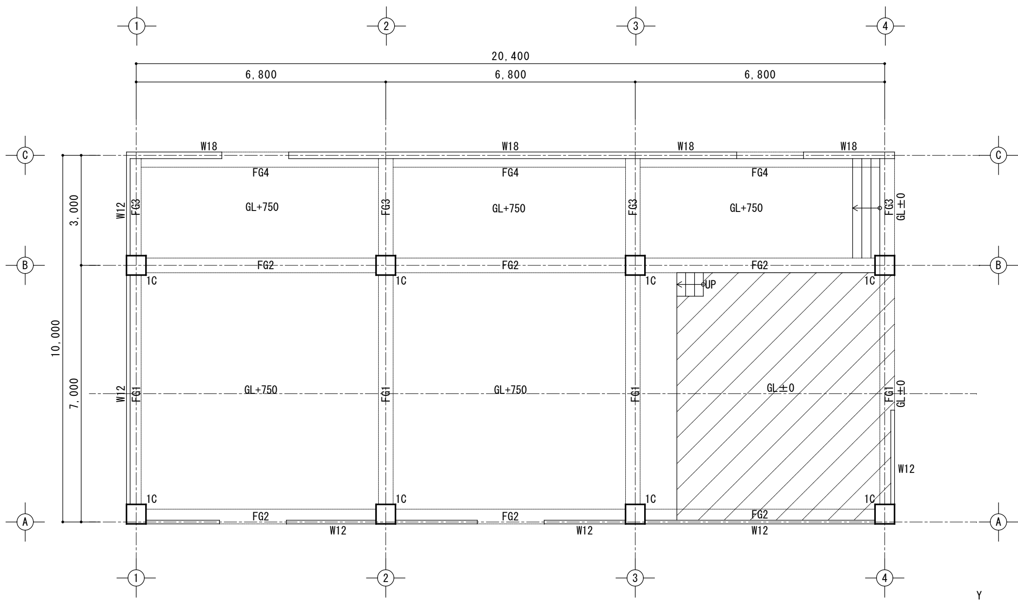
1 階 伏 図 1/100
