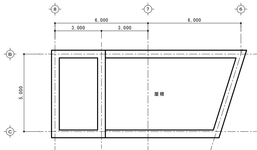
屋上 平面図
