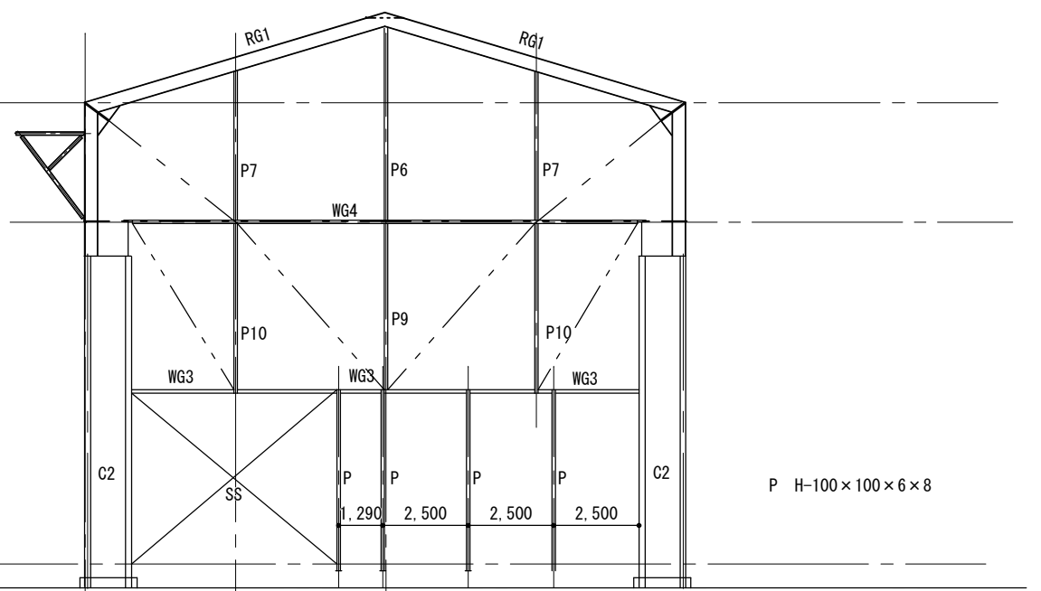
⑮ 通り軸組図 S:1/200
