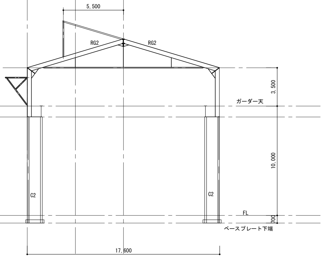
⑮ 通り軸組図 S:1/200
