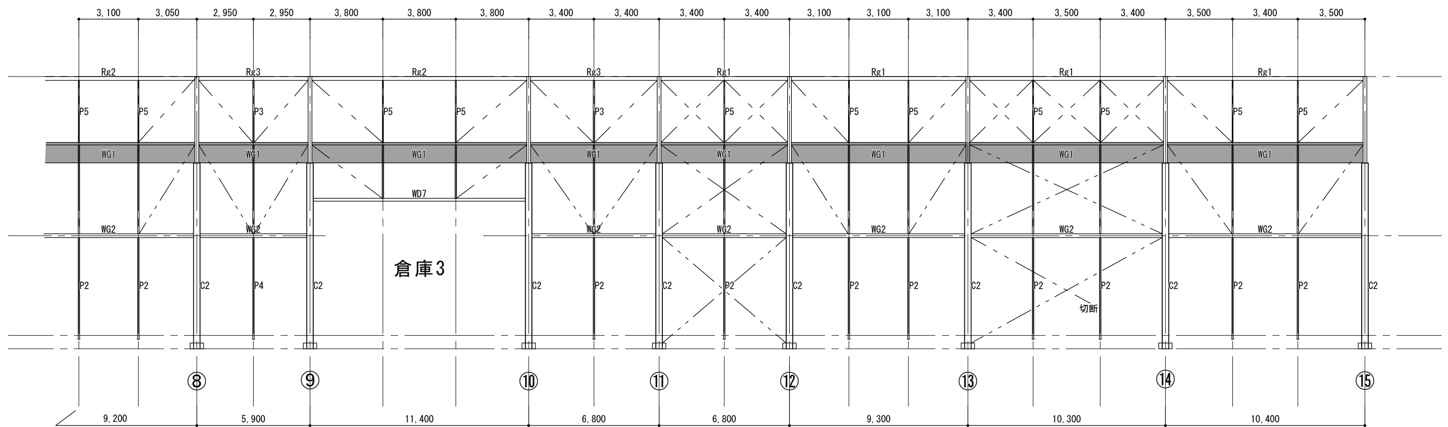
A通り軸組図 S:1/200
