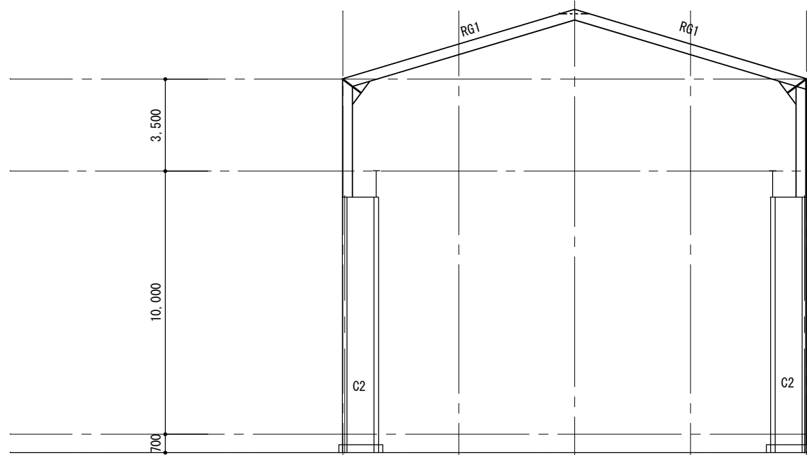
④ 通り軸組図 S:1/200
