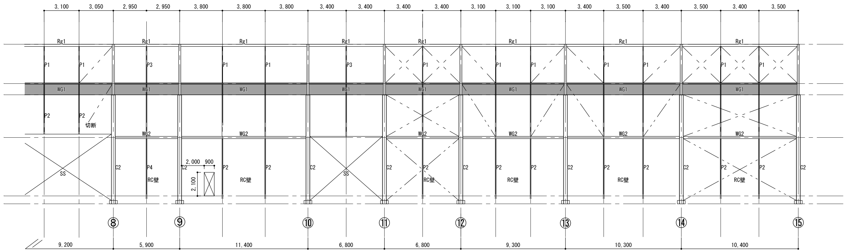
B通り軸組図 S:1/200
