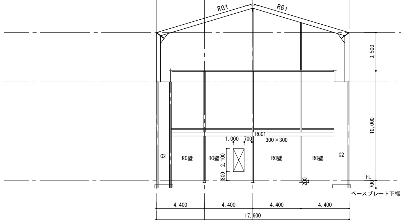
① 通り軸組図 S:1/200
