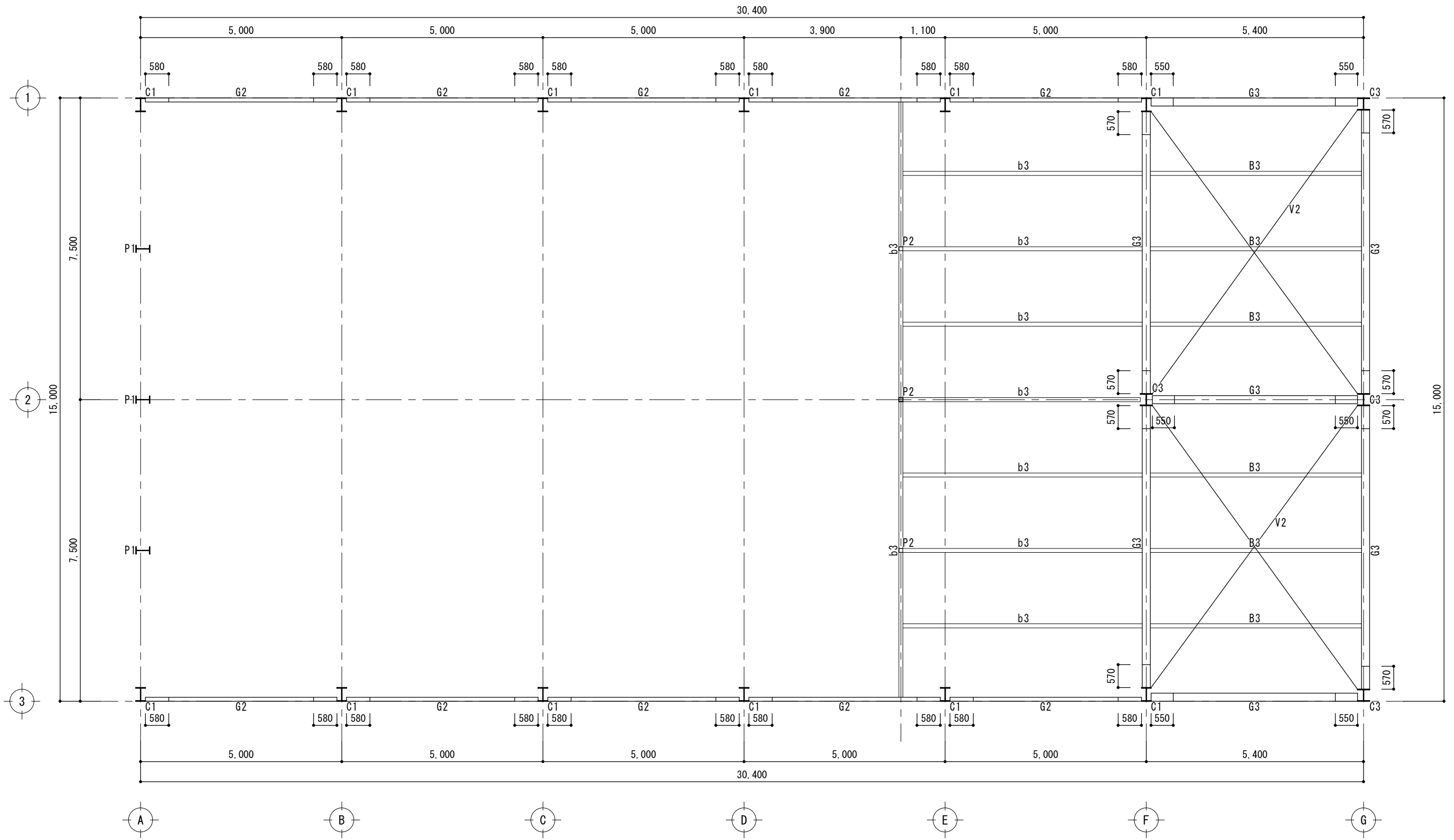
小屋伏図
