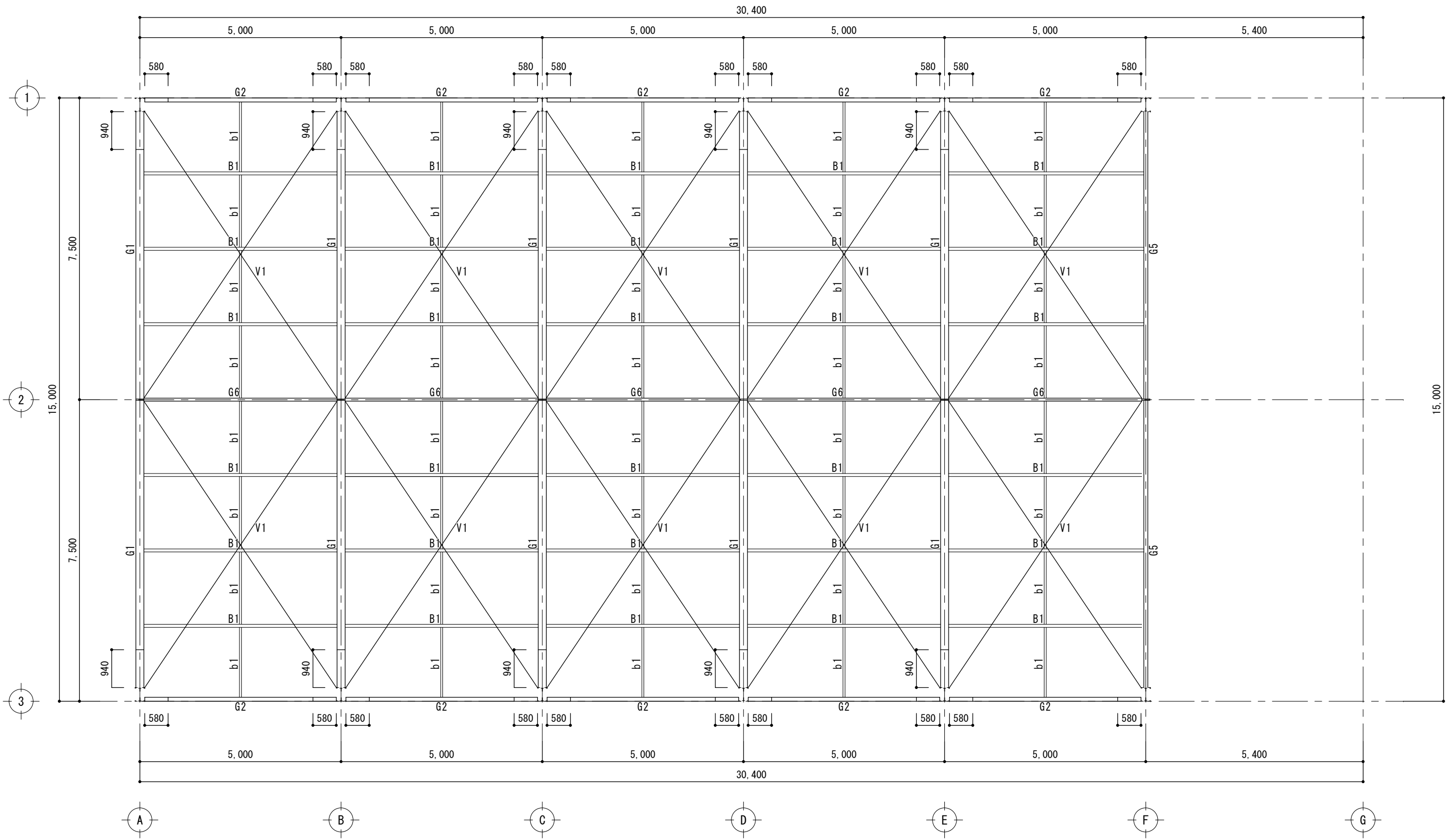
屋根伏図
