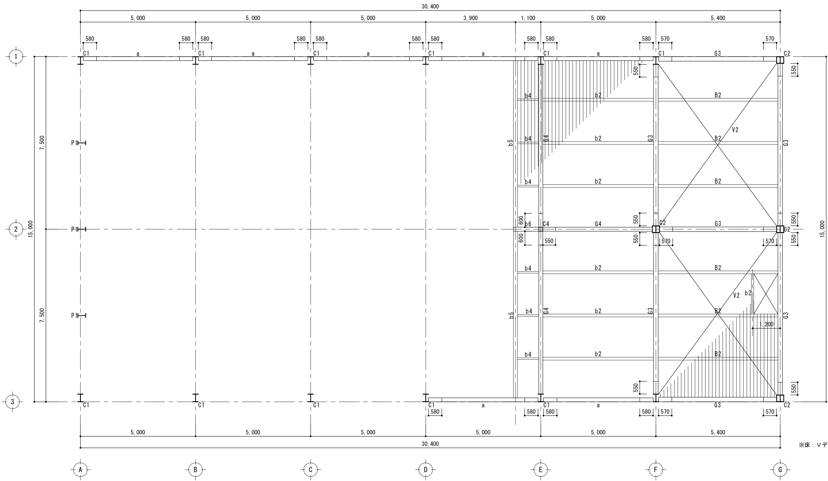
2階床伏図
