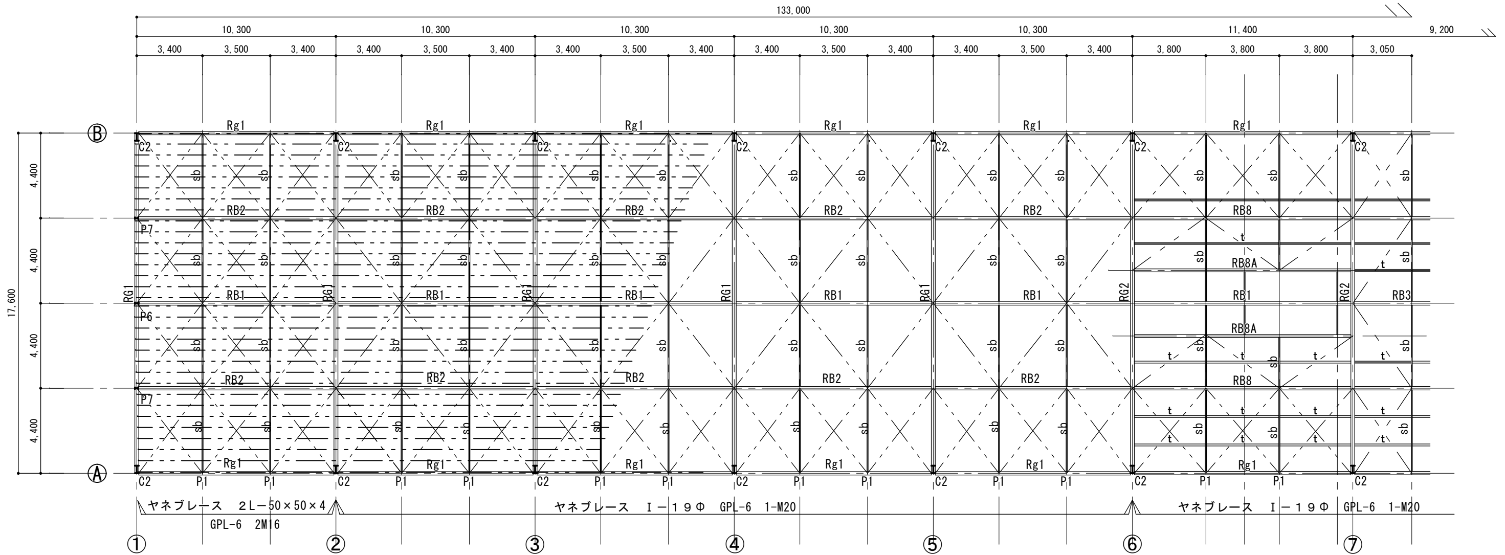
小屋伏図 S:1/200
