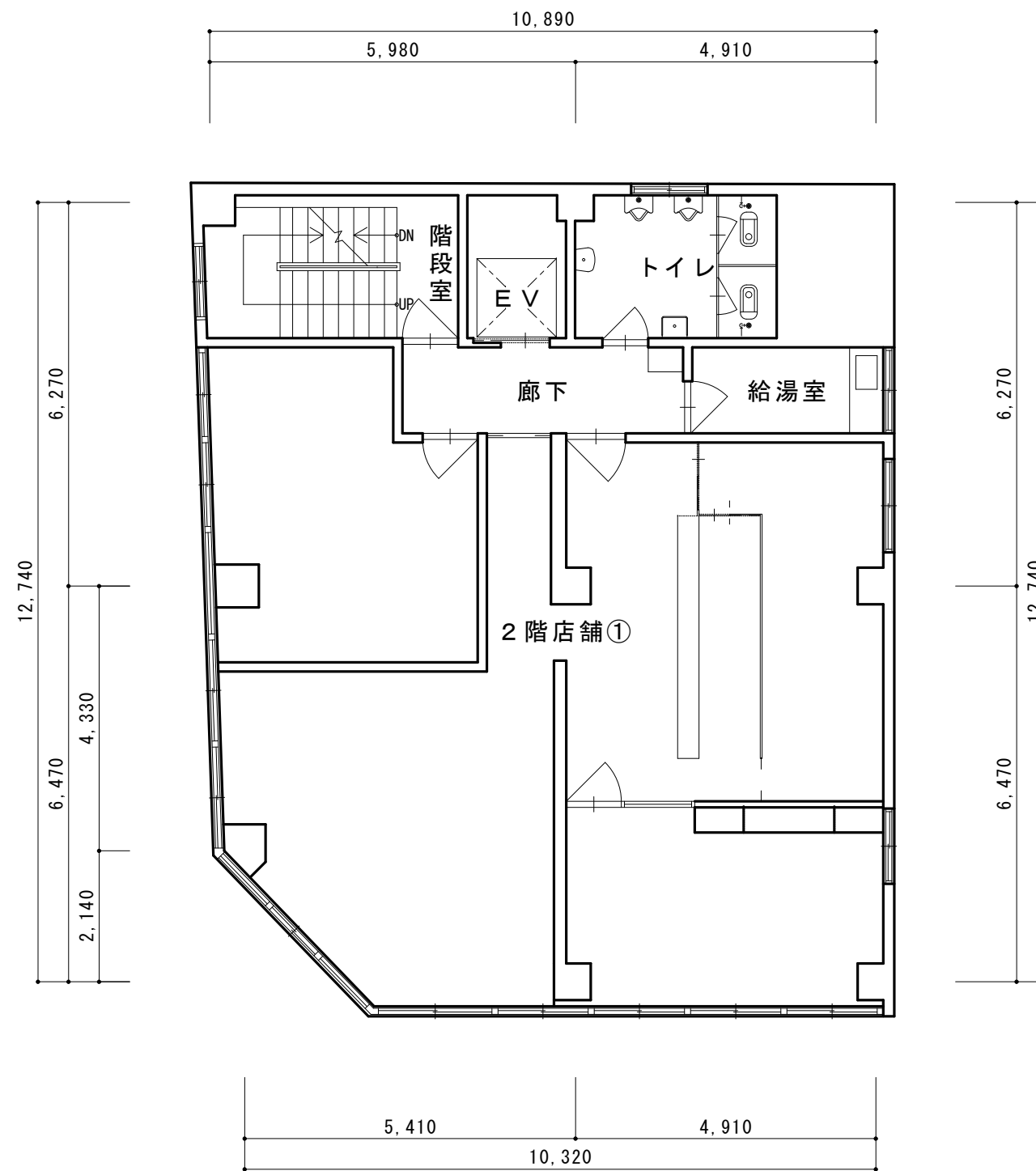
2 F 平面図
