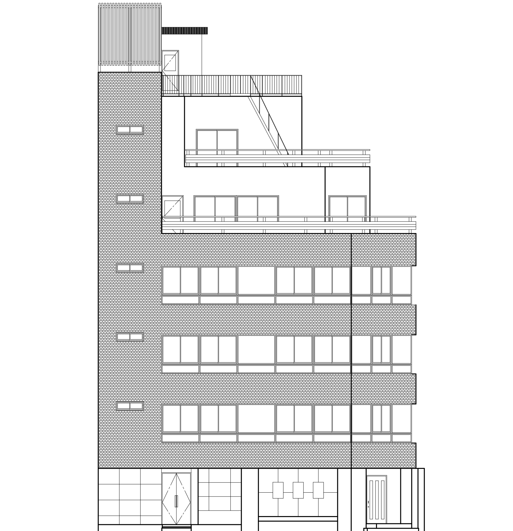
西立面图
