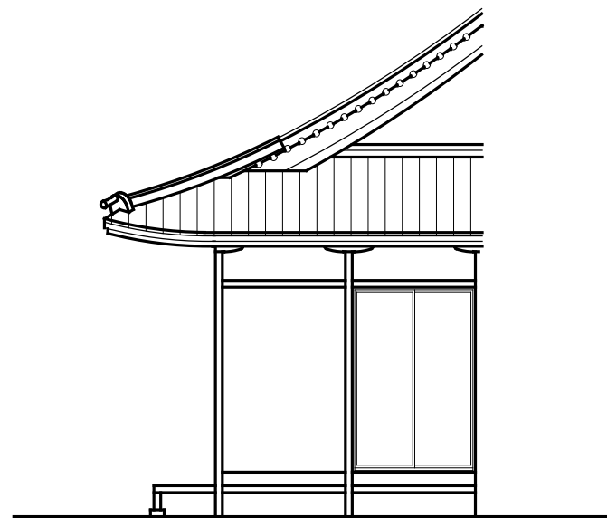
北立面図 S=1/100
