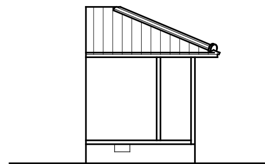
南立面図 S=1/100
