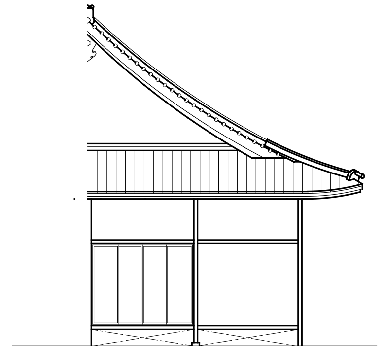
北立面图 S=1/100
