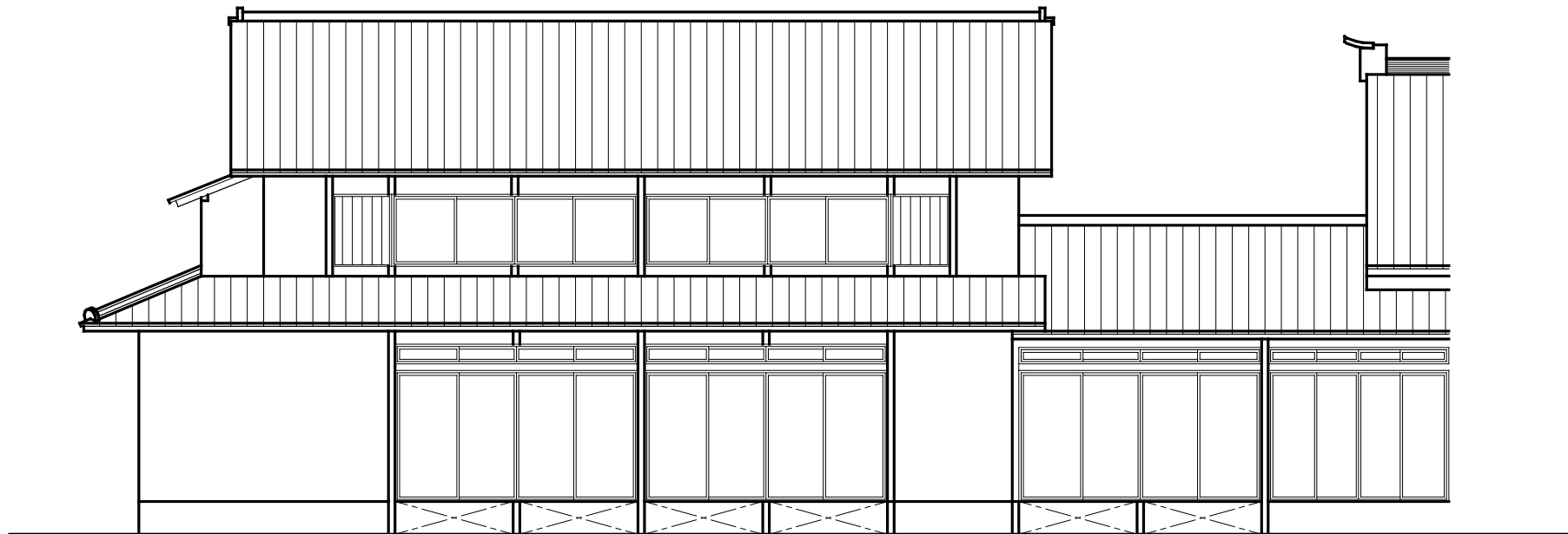
南立面图 S=1/100
