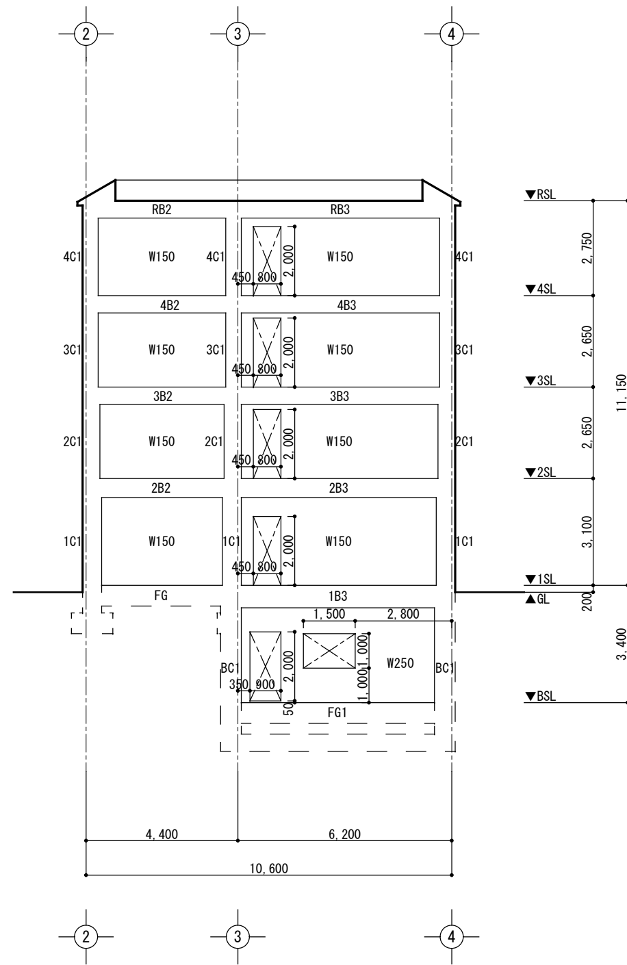
A通 軸組図 1/150
