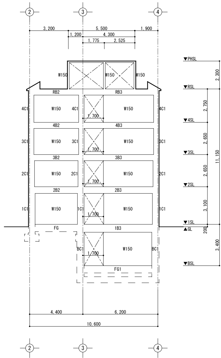
B通 軸組図 1/150
