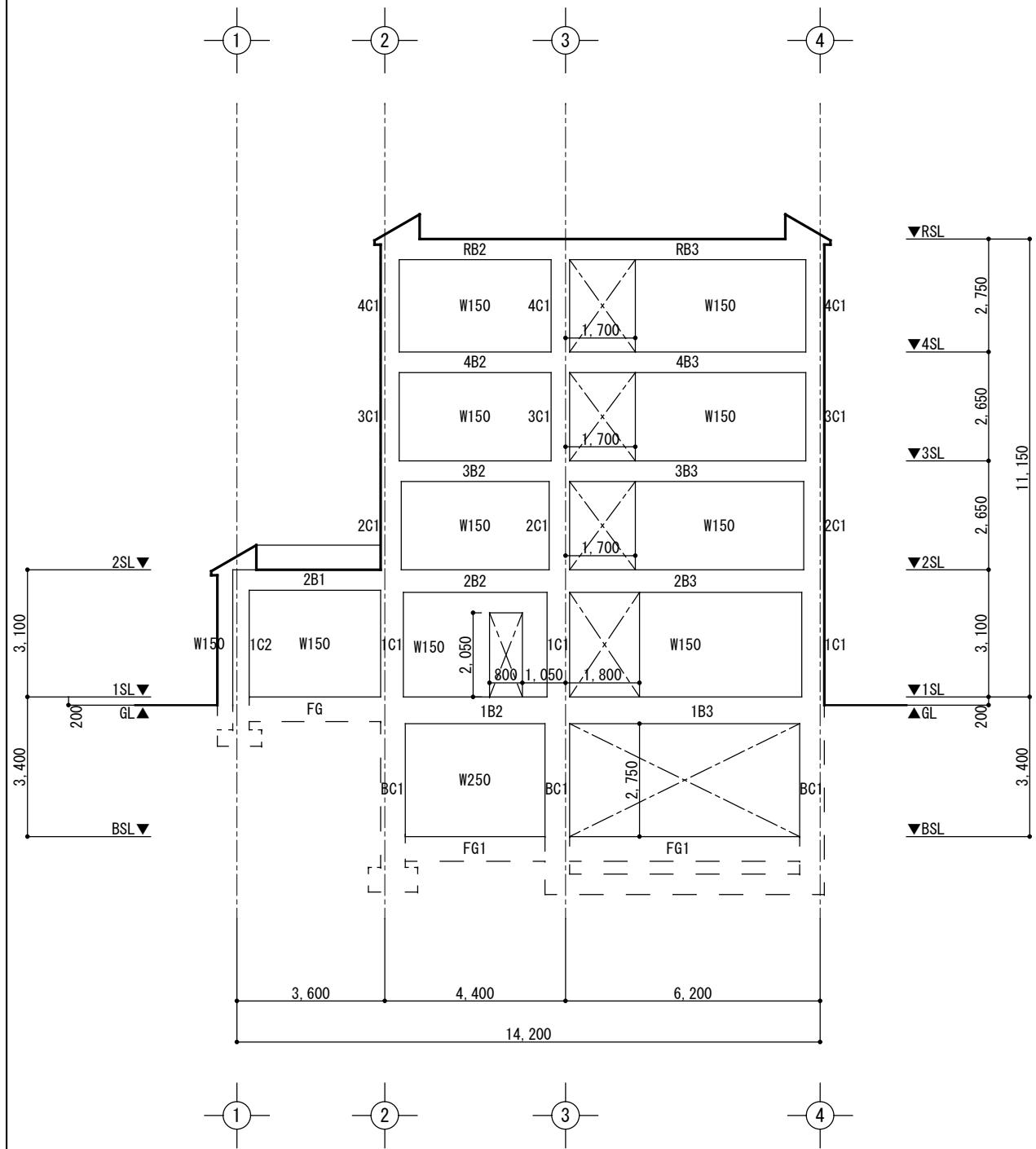
C通軸組図 1/150
