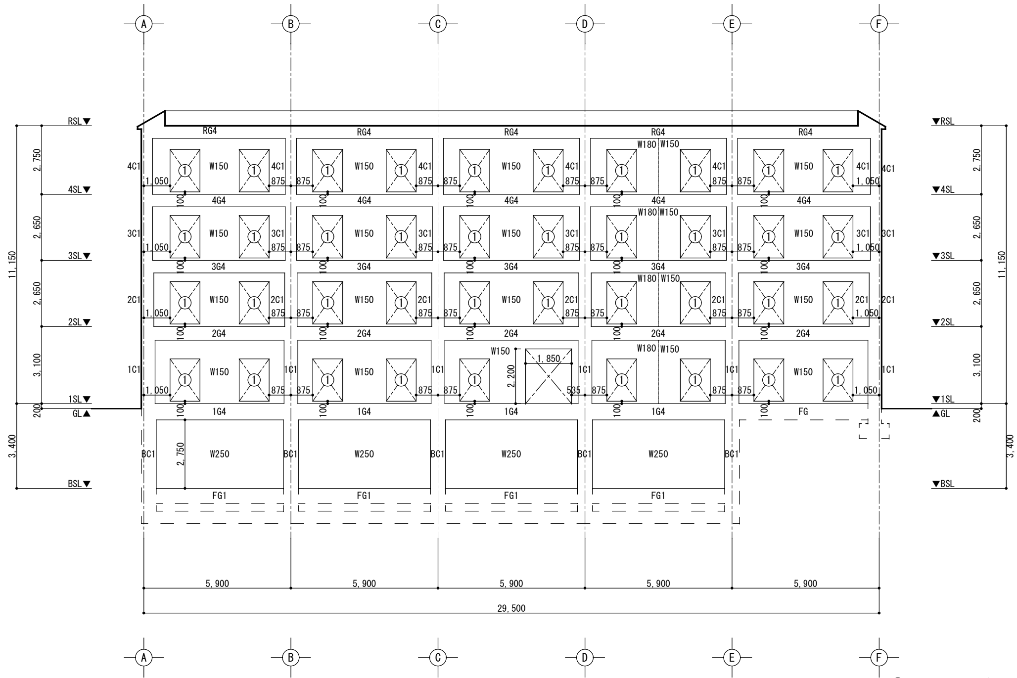
4通 軸組図 1/150
