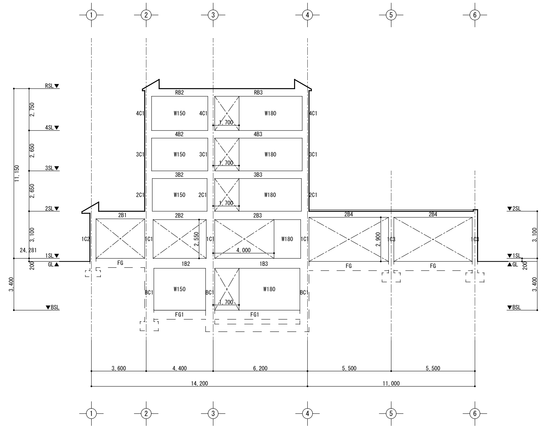
D通軸組図 1/150
