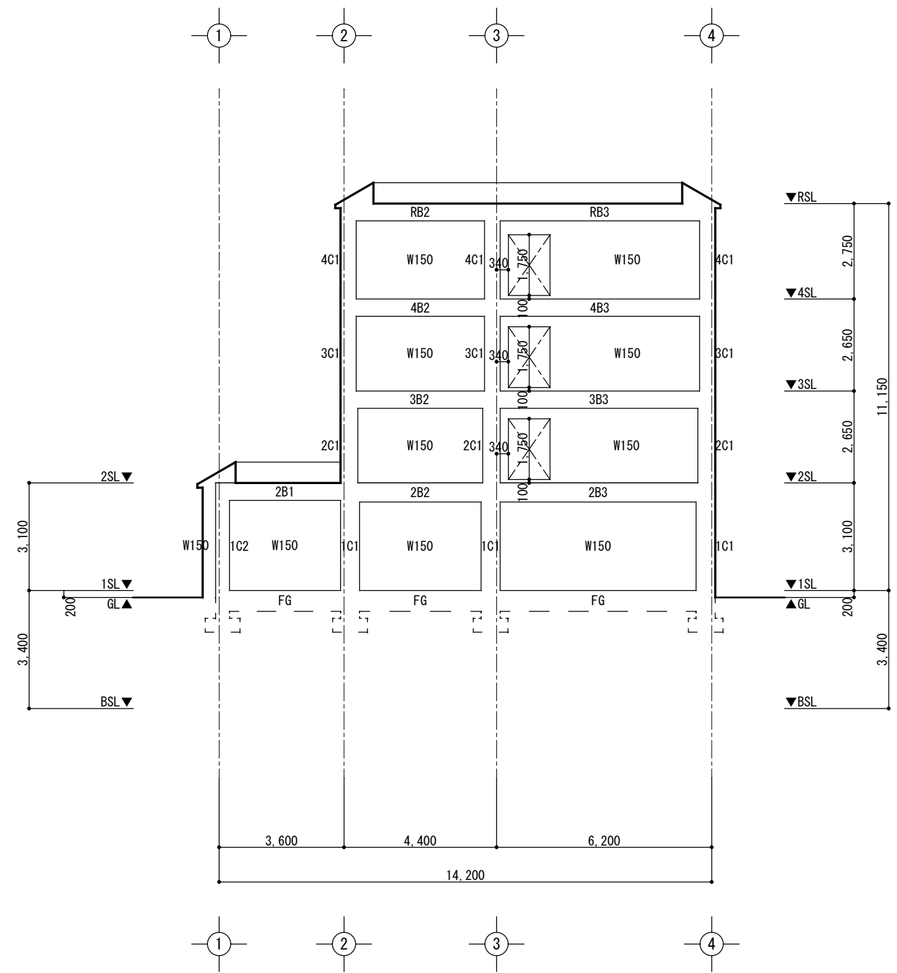
F通 軸組図 1/150
