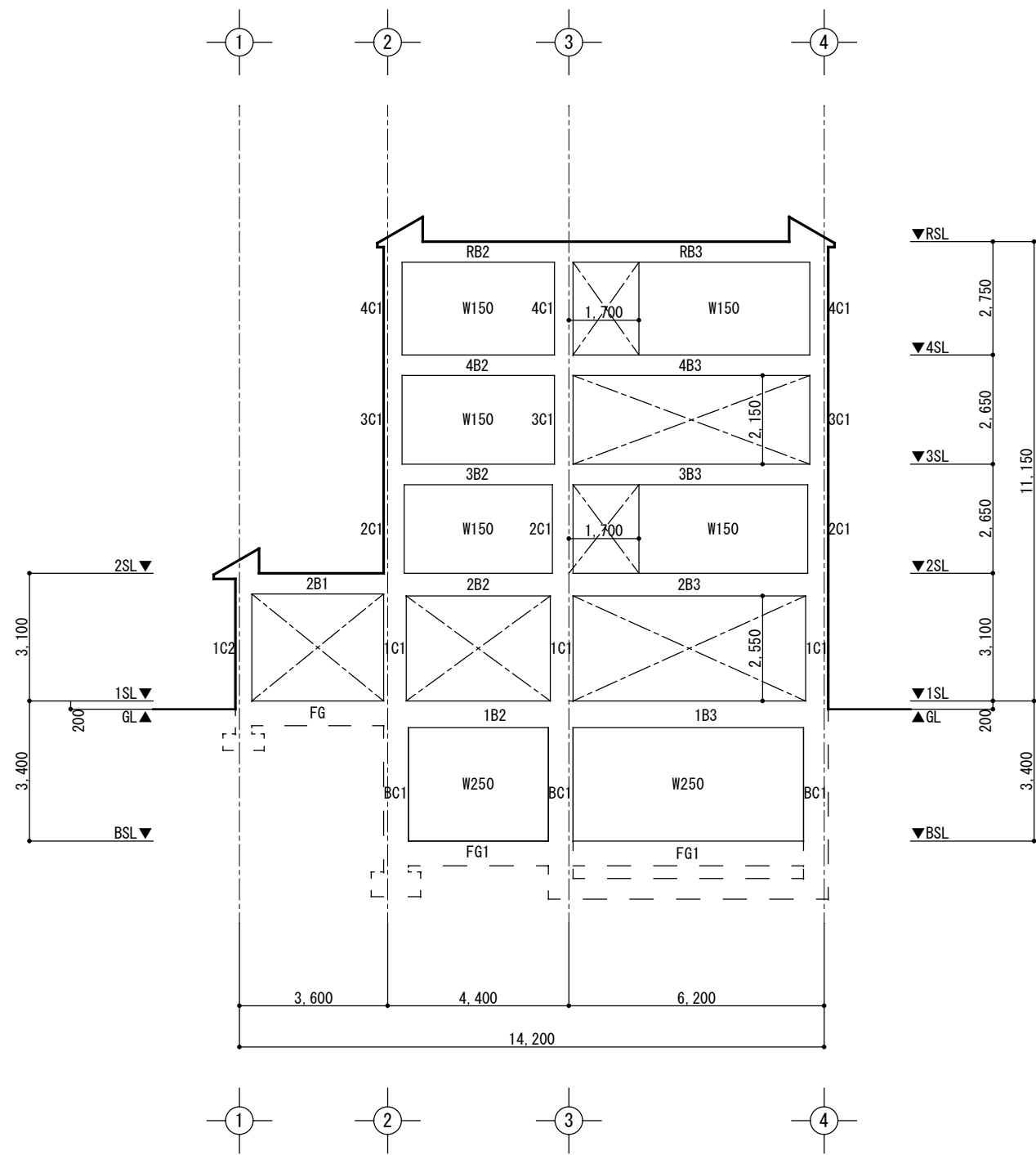
E通 軸組図 1/150
