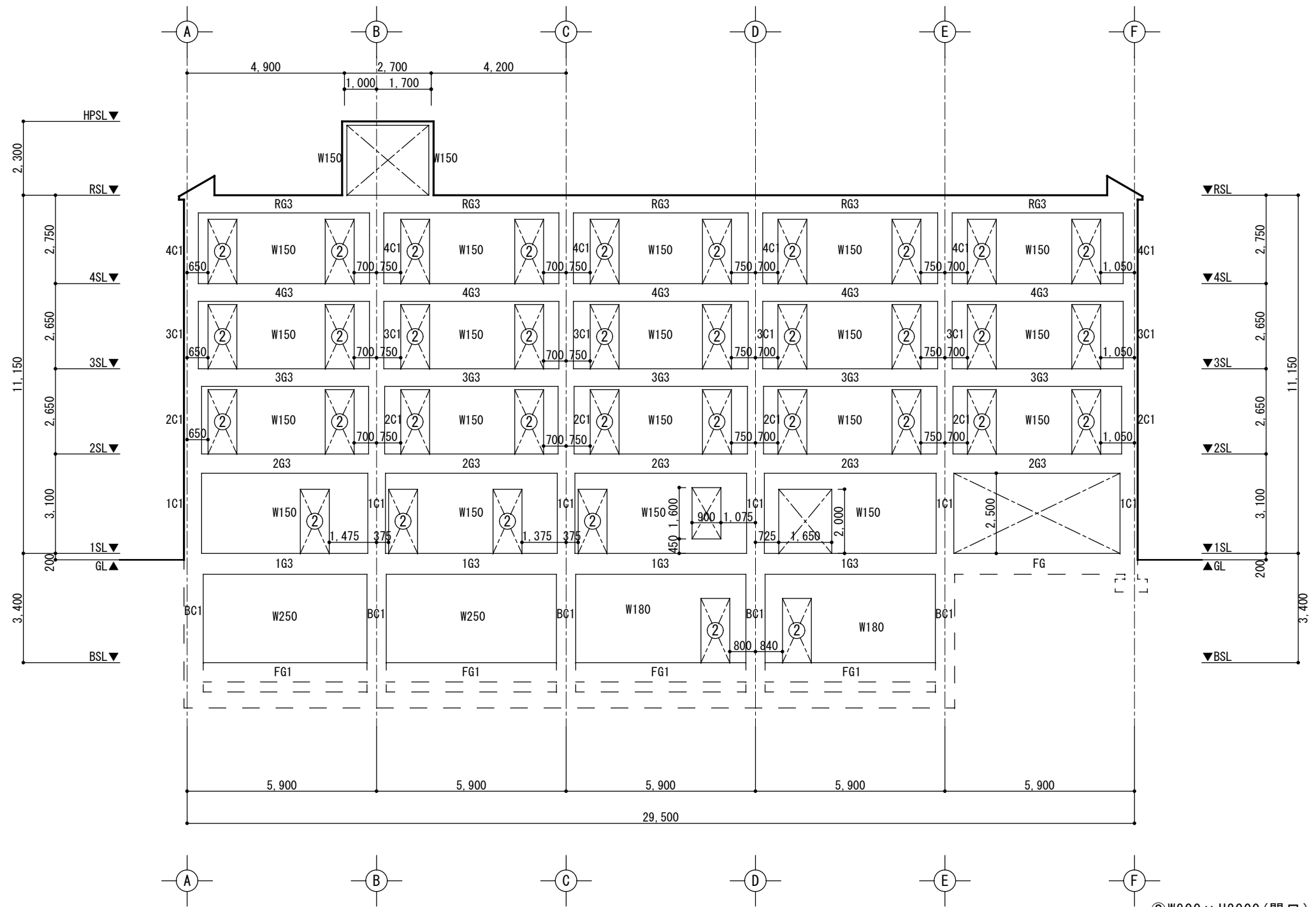
3通 軸組図 1/150
