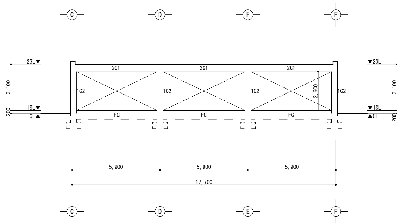
1通 軸組図 1/150
