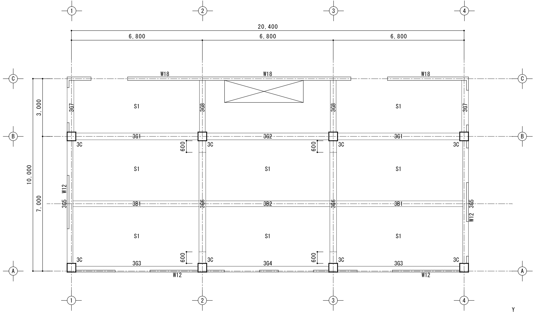
3階伏図 1/100
