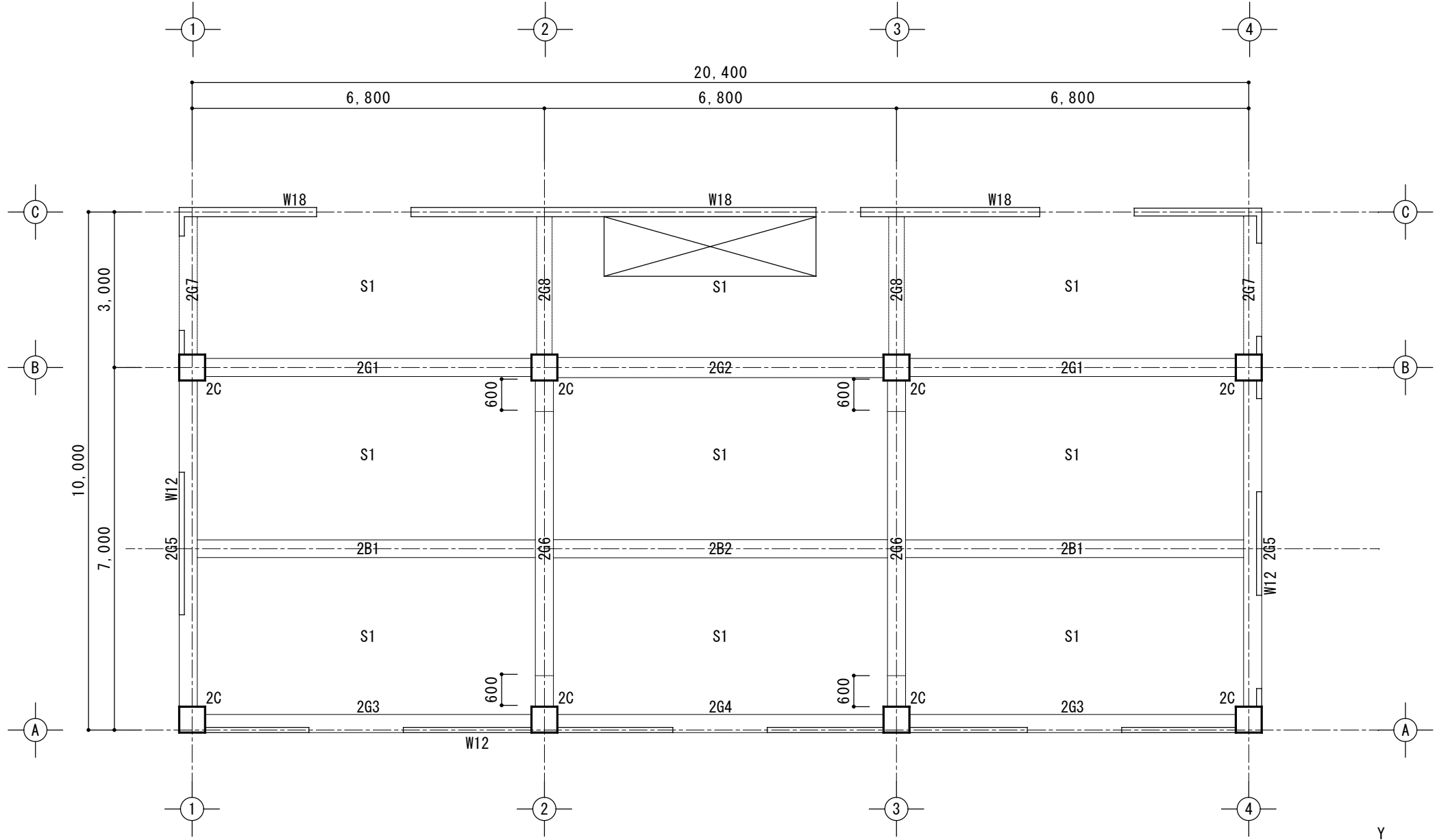
2階伏図 1/100
