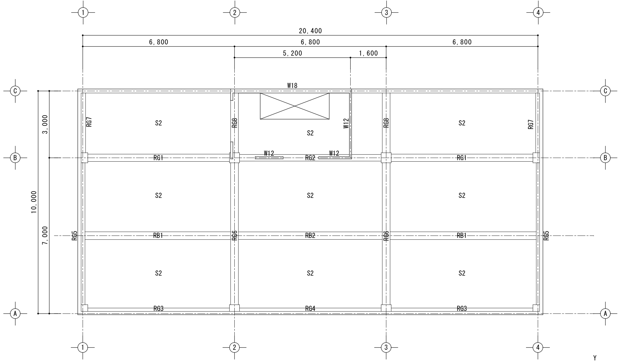
R 階伏図 1/100
