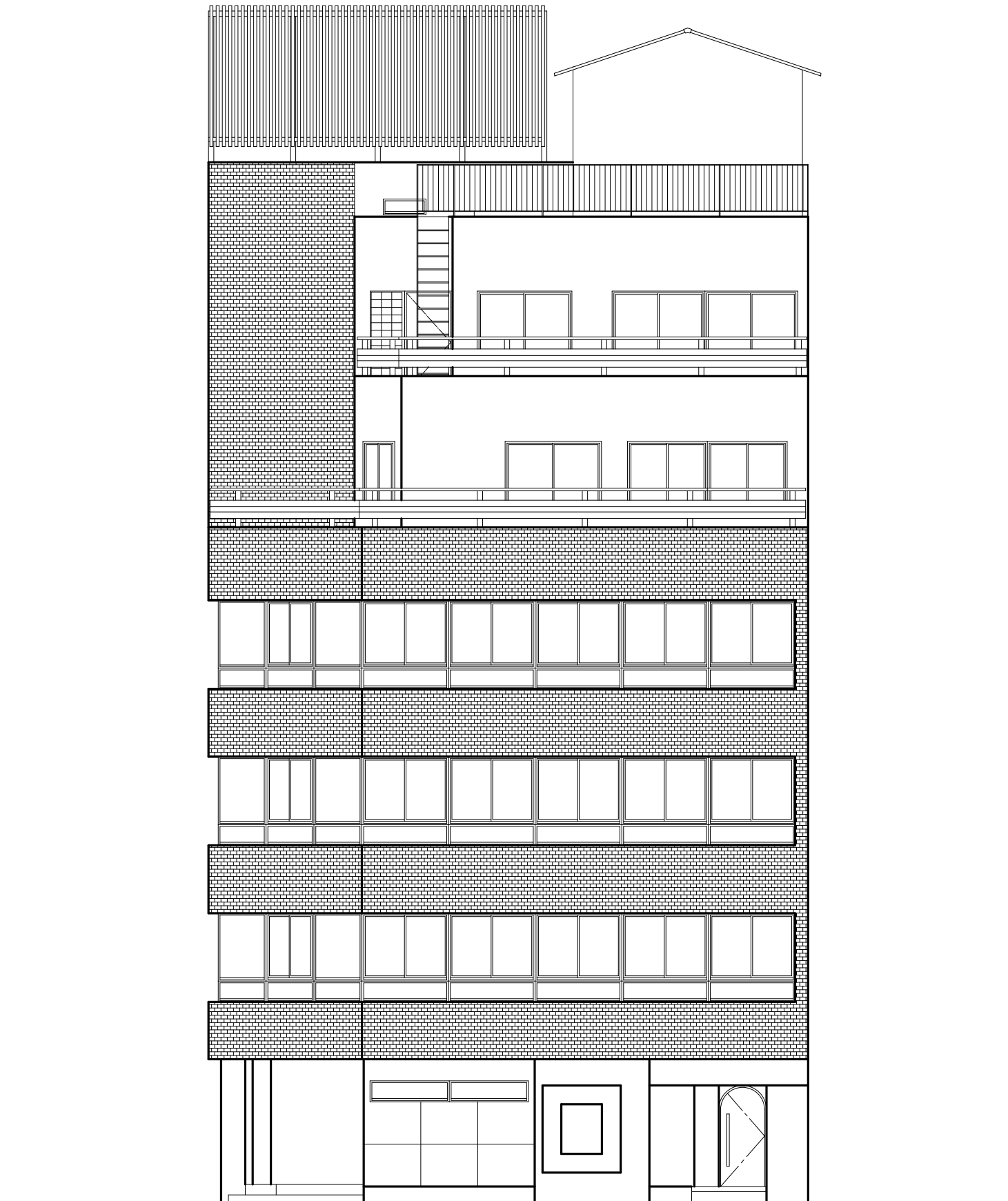
南立面图
