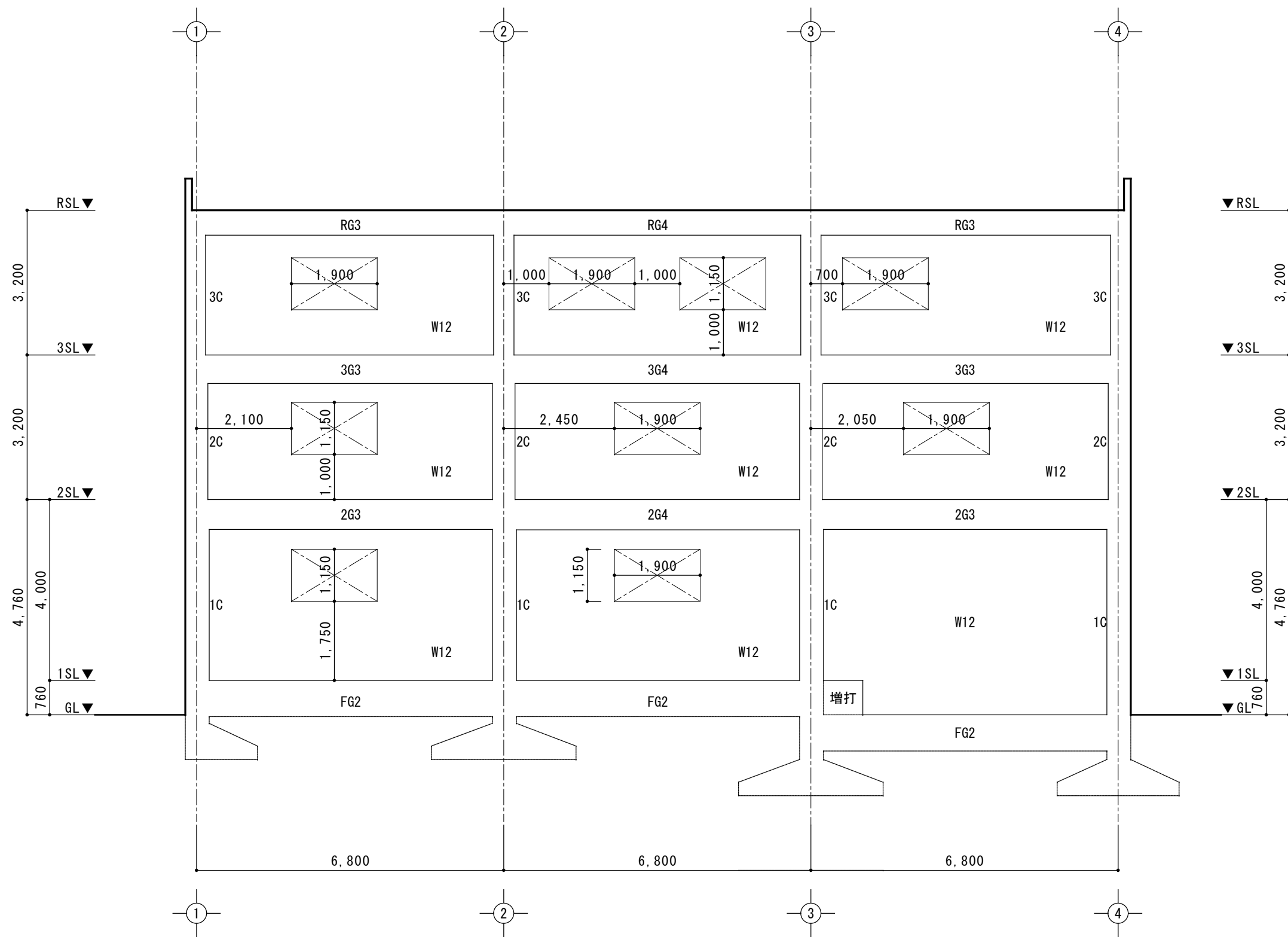
A通 軸組図 1/100
