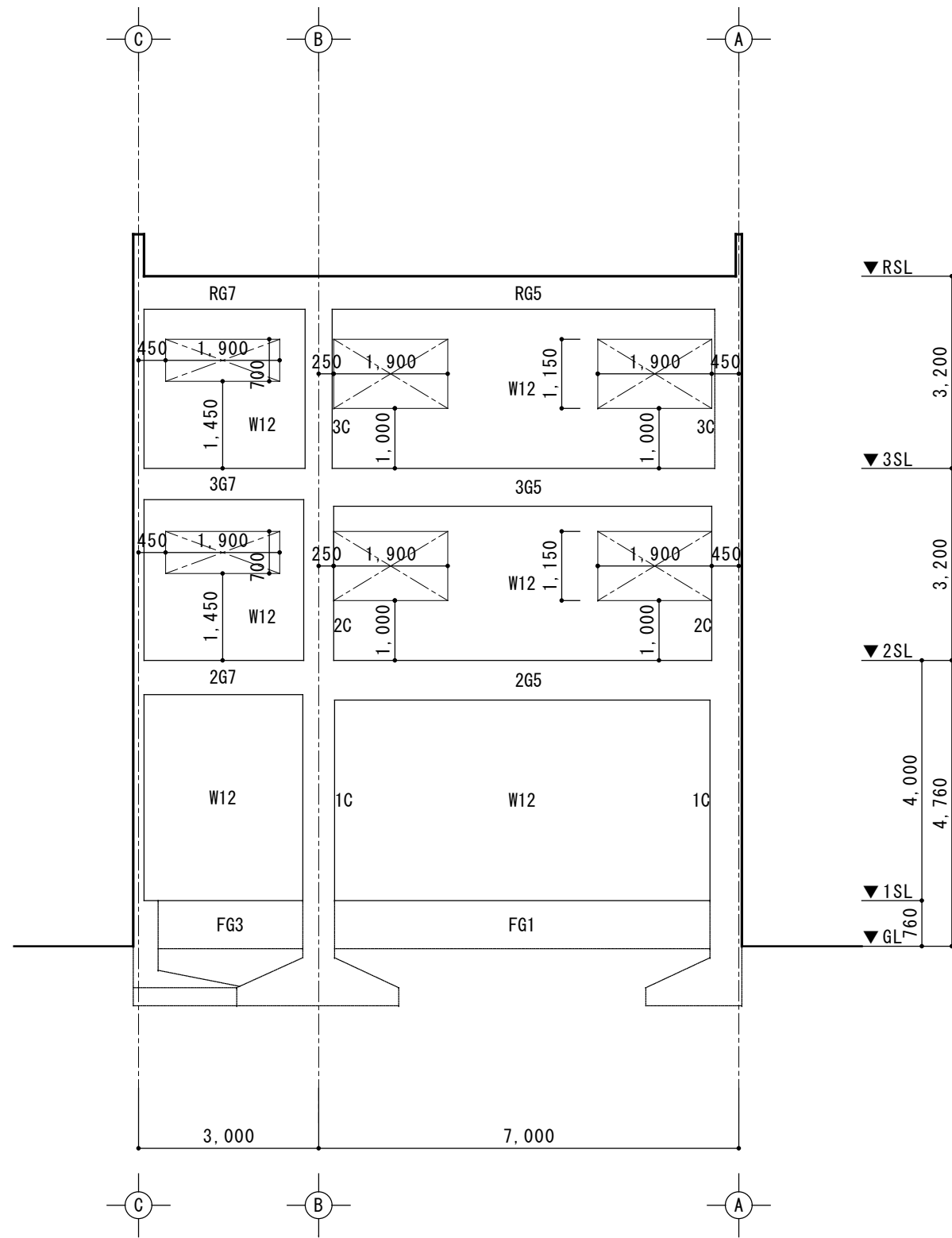
1通 軸組図 1/100
