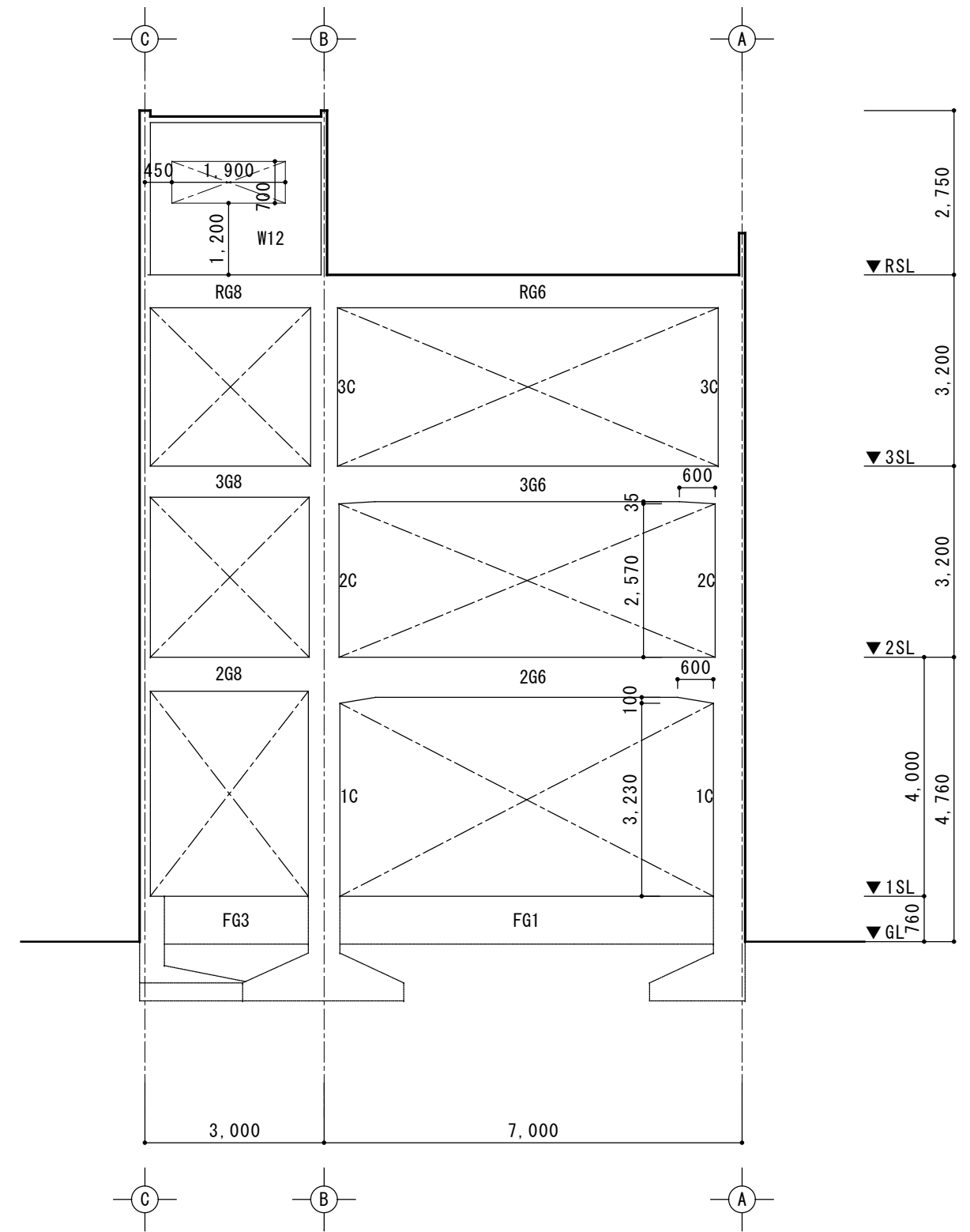
2通 軸組図 1/100
