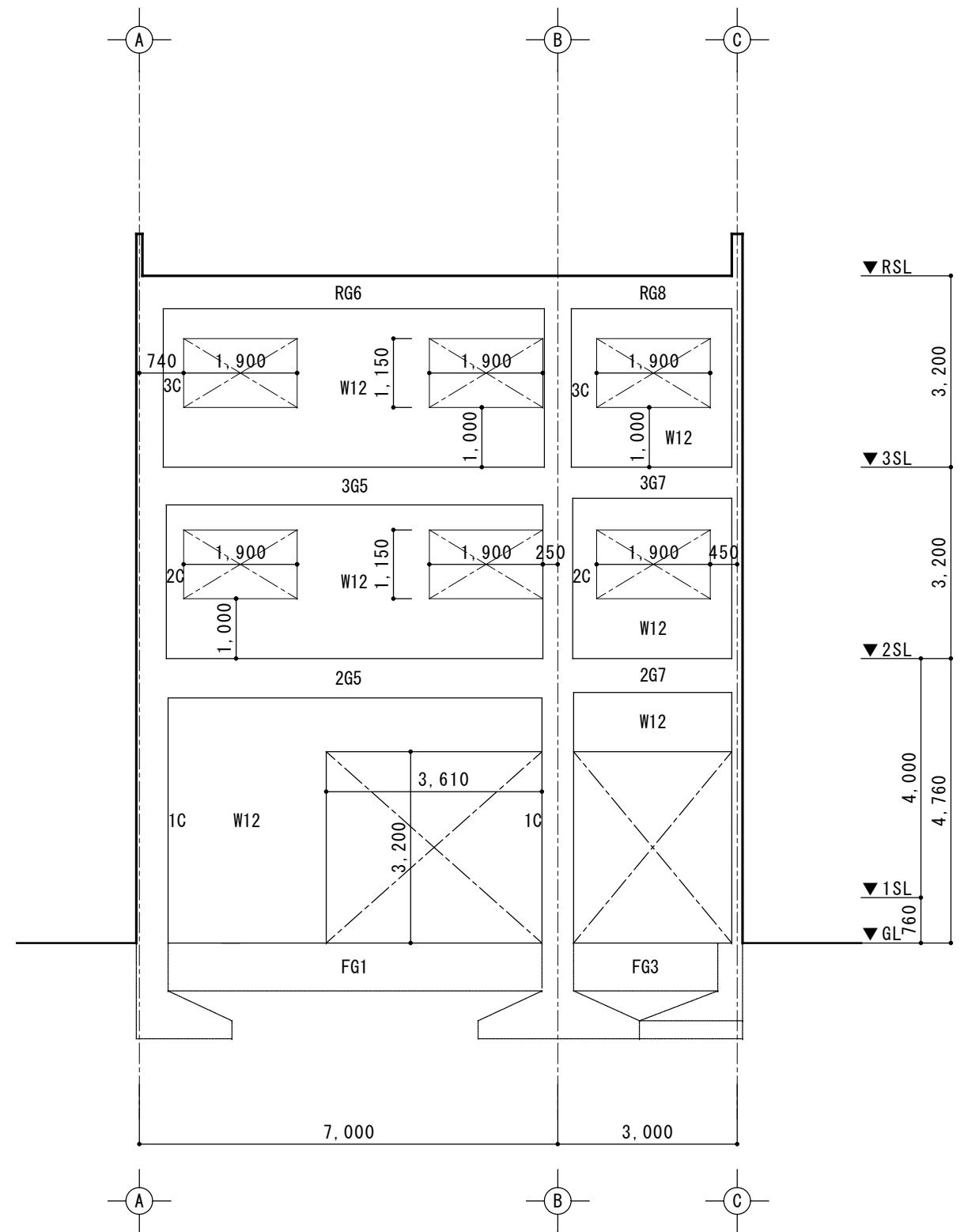
4通 軸組図 1/100
