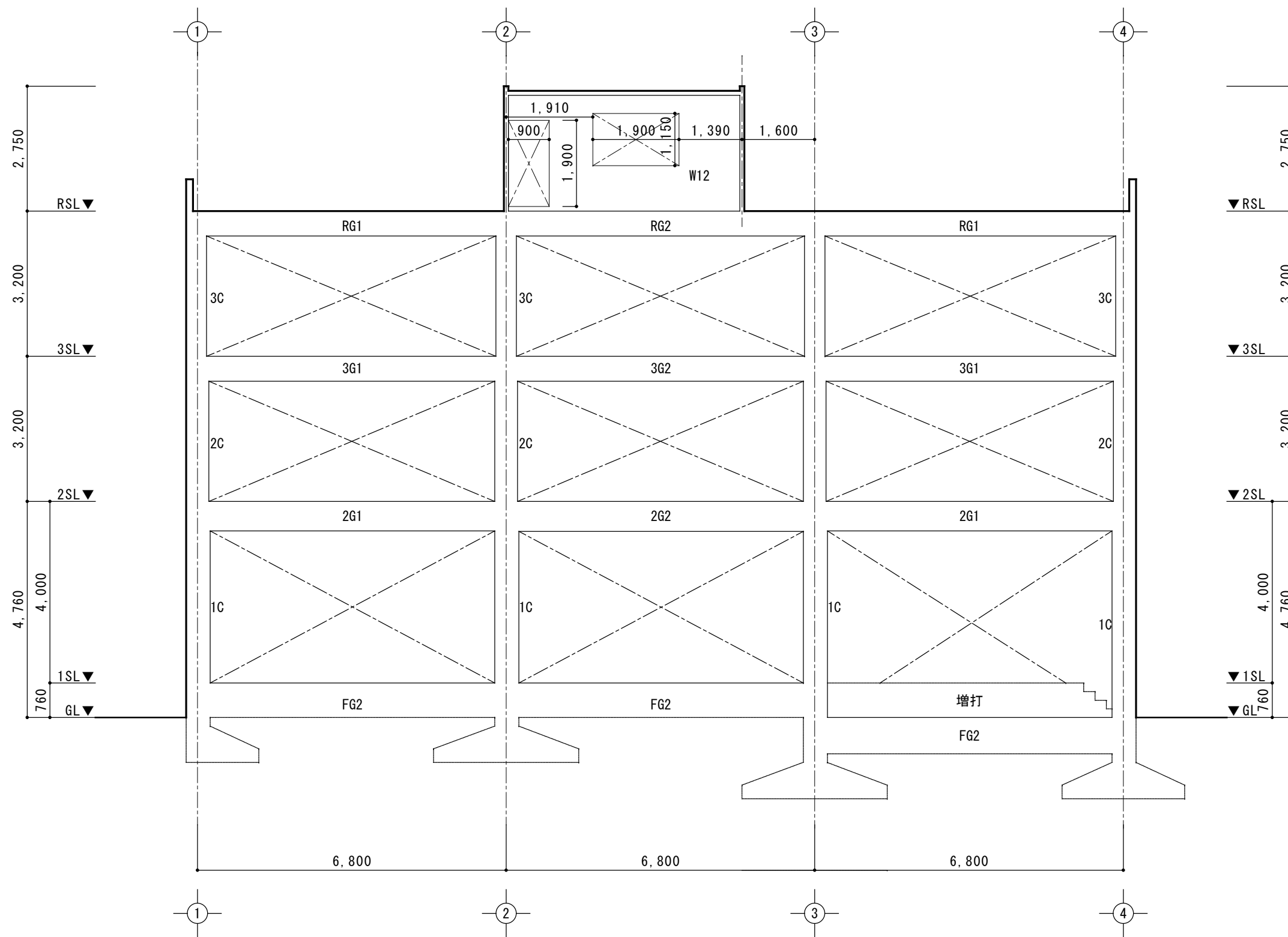
B通 軸組図 1/100
