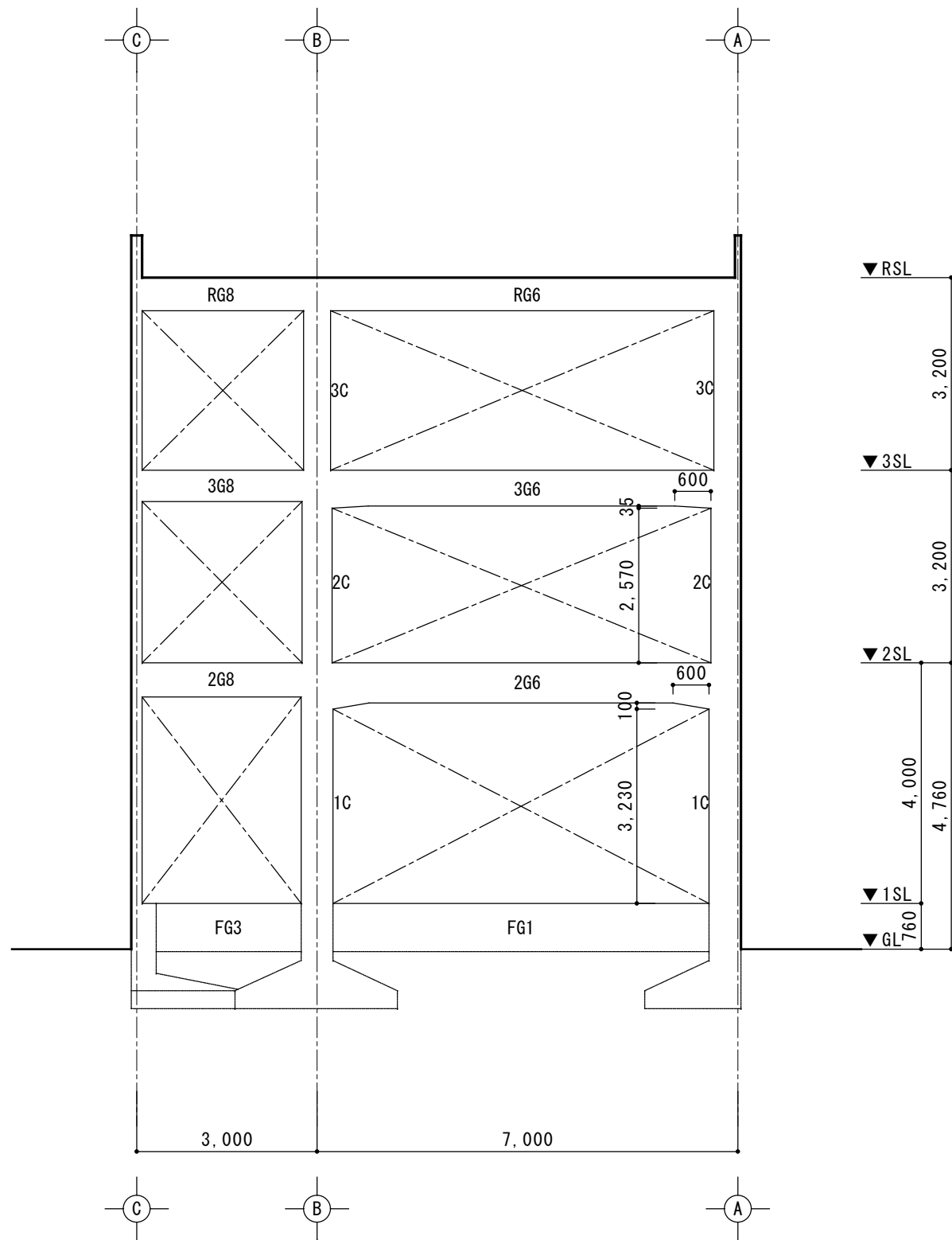
3通 軸組図 1/100
